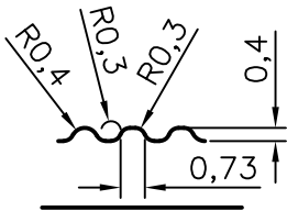
Detalle A Esc.: 4:1
